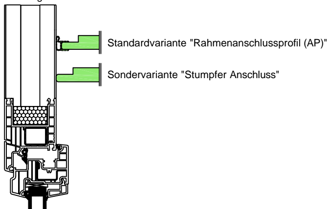
Vorhangbrett-Rahmenanschluss-Varianten
