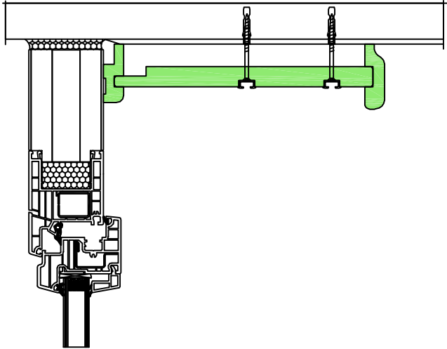
Vorhangbrett Wetraform STA, Standardmontage
