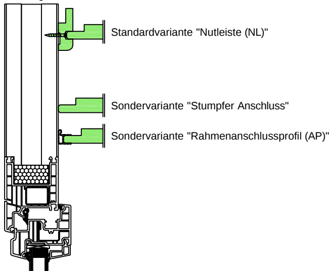
Vorhangbrett-Rahmenanschluss-Varianten
