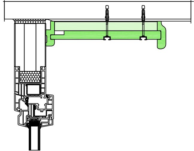
Vorhangbrett Wetraform STA, mit Isolationsauflage 20 mm
